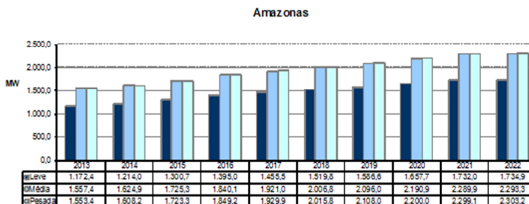
Gráfico 62 – Evolução da carga do Estado do Amazonas
