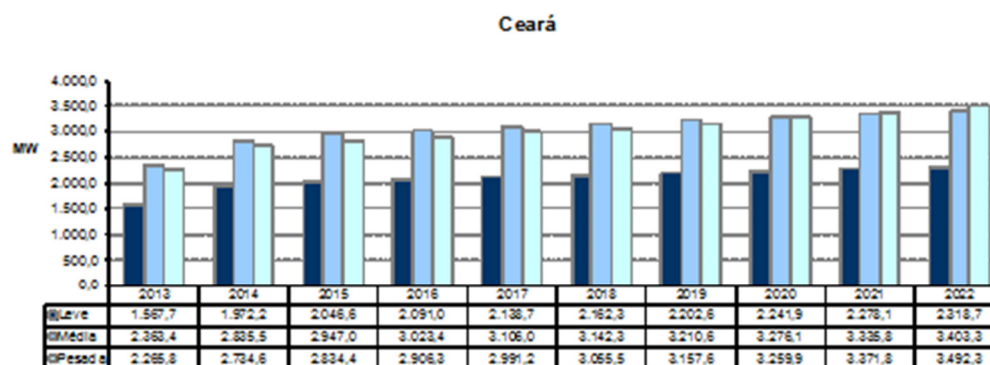
Gráfico 67 – Evolução da carga do Estado do Ceará
