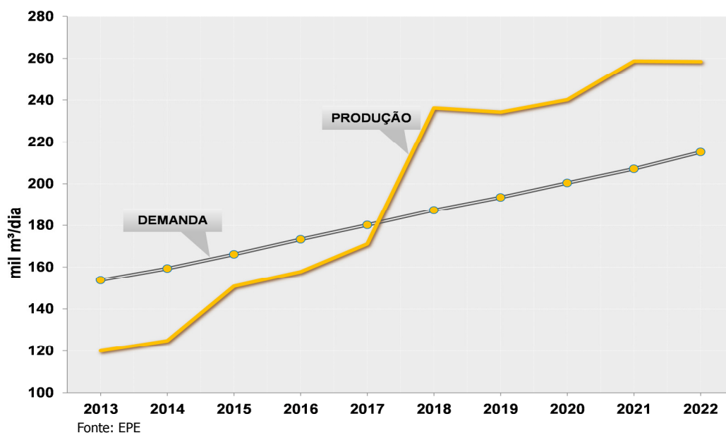
Gráfico 114 – Balanço de diesel
