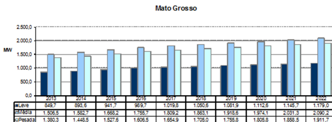
Gráfico 81 – Evolução da carga de Estado de Mato Grosso
