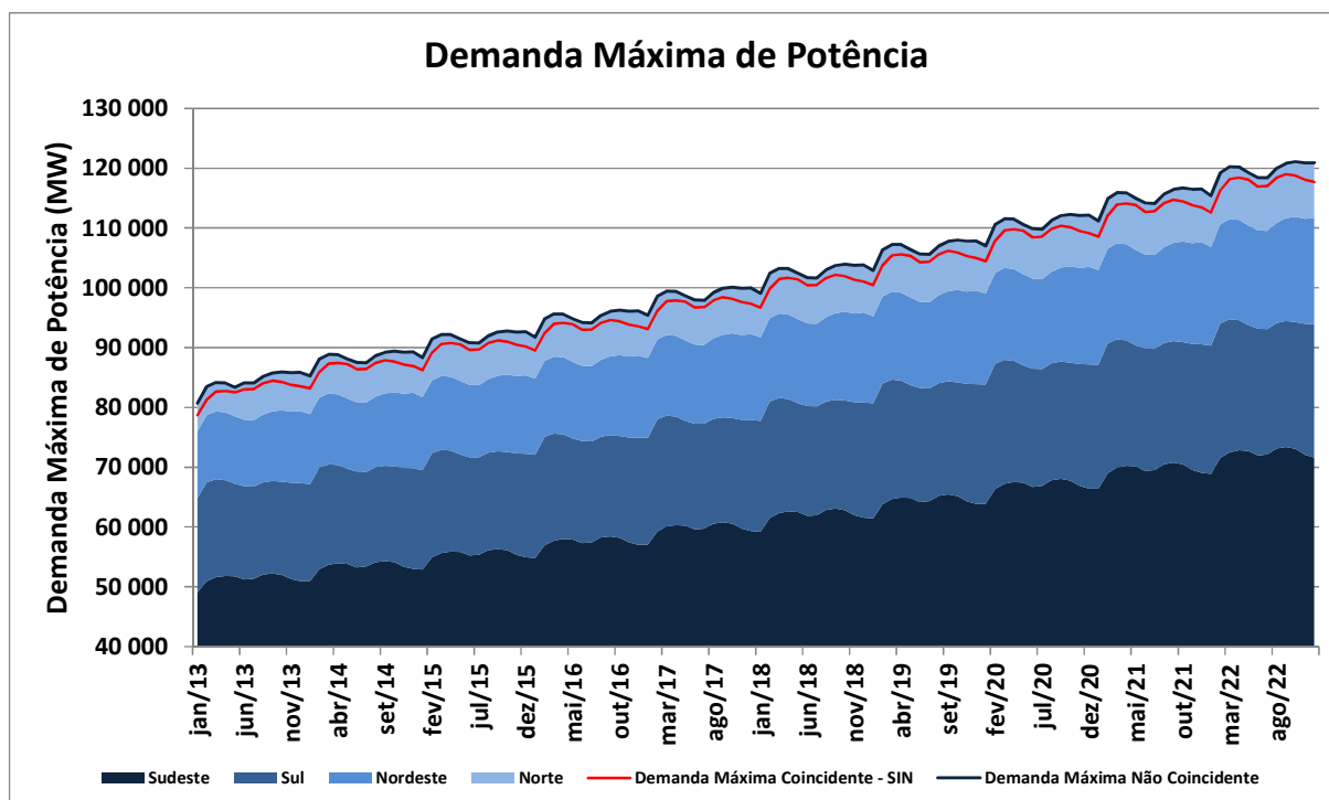
Gráfico 47 – Comparação entre demanda máxima coincidente e não-coincidente
