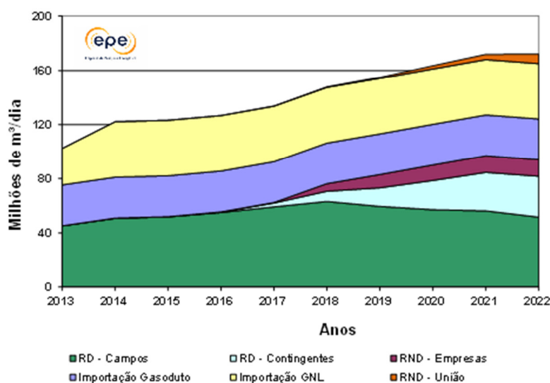
Gráfico 123 – Oferta total Brasil (malha integrada)
