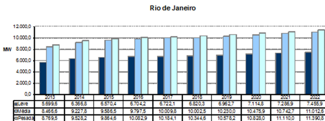
Gráfico 78 – Evolução da carga do Estado do Rio de Janeiro
