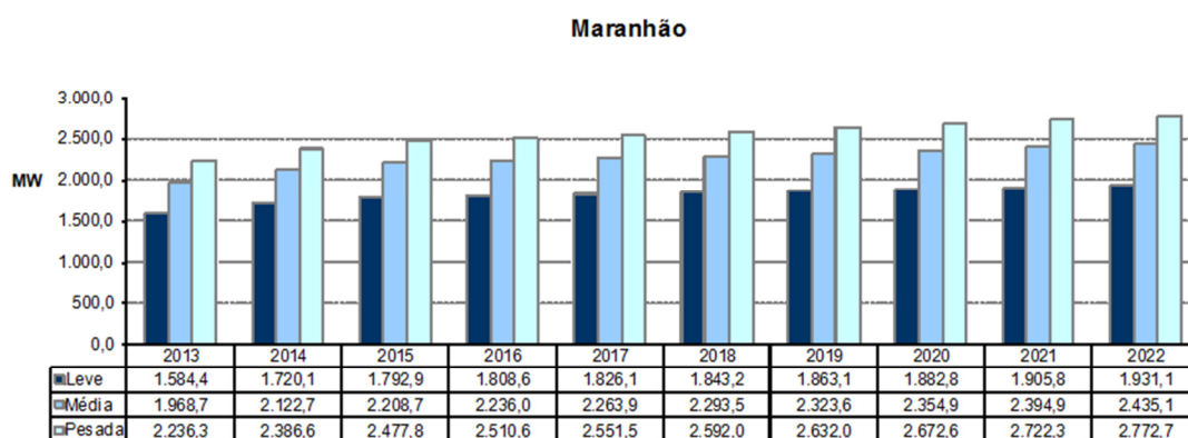
Gráfico 60 – Evolução da carga do Estado do Maranhão
