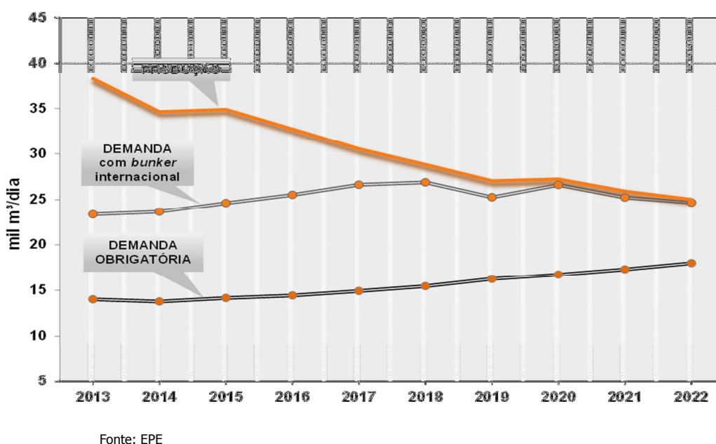
Gráfico 115 – Balanço de óleo combustível
