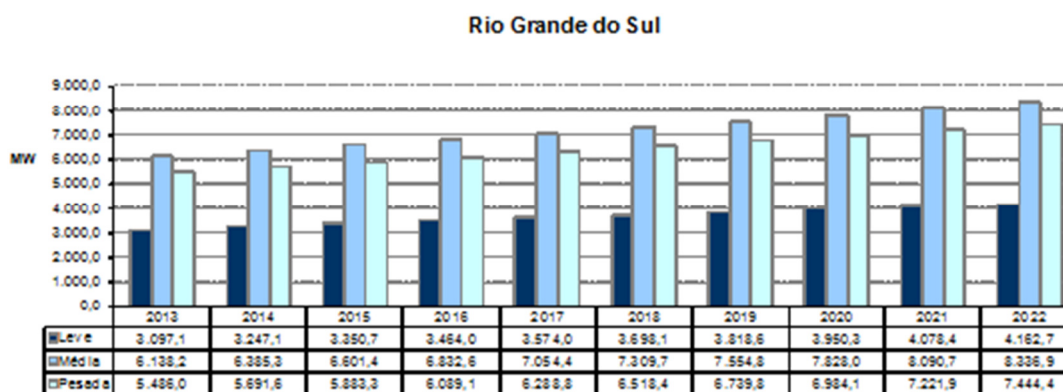
Gráfico 84 – Evolução da carga do Estado do Rio Grande do Sul
