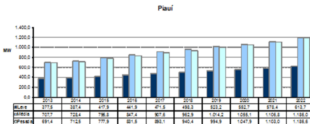
Gráfico 66 – Evolução da carga do Estado do Piauí
