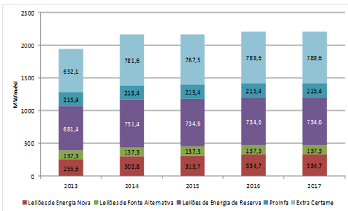
Gráfico 136 – Energia contratada nos Leilões de Energia e extra certame
