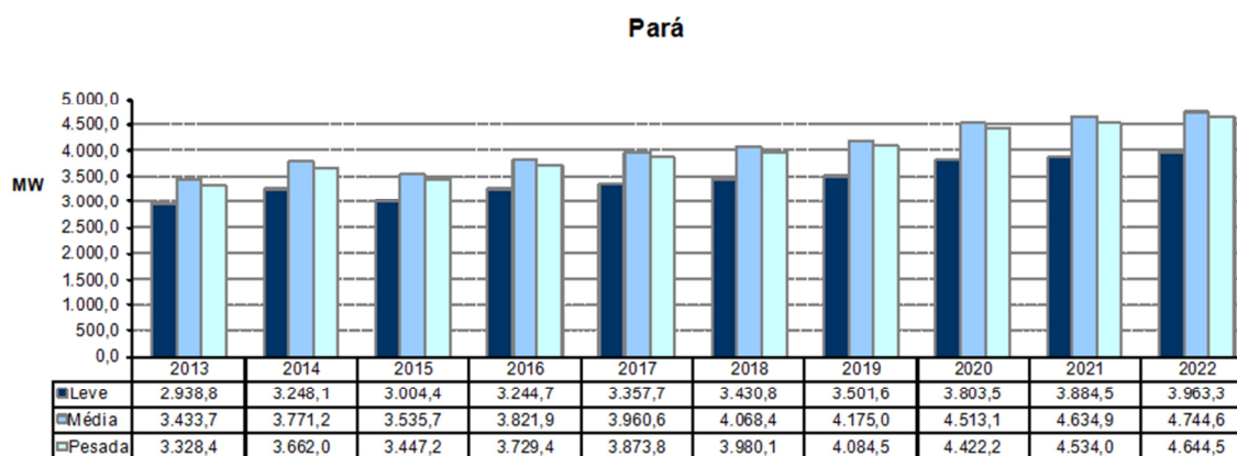
Gráfico 59 – Evolução da carga do Estado do Pará
