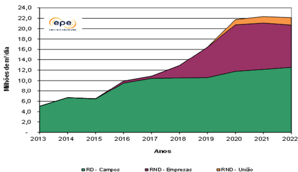
Gráfico 120 – Oferta total da Região Norte
