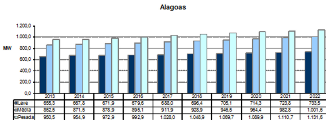
Gráfico 71 – Evolução da carga do Estado de Alagoas
