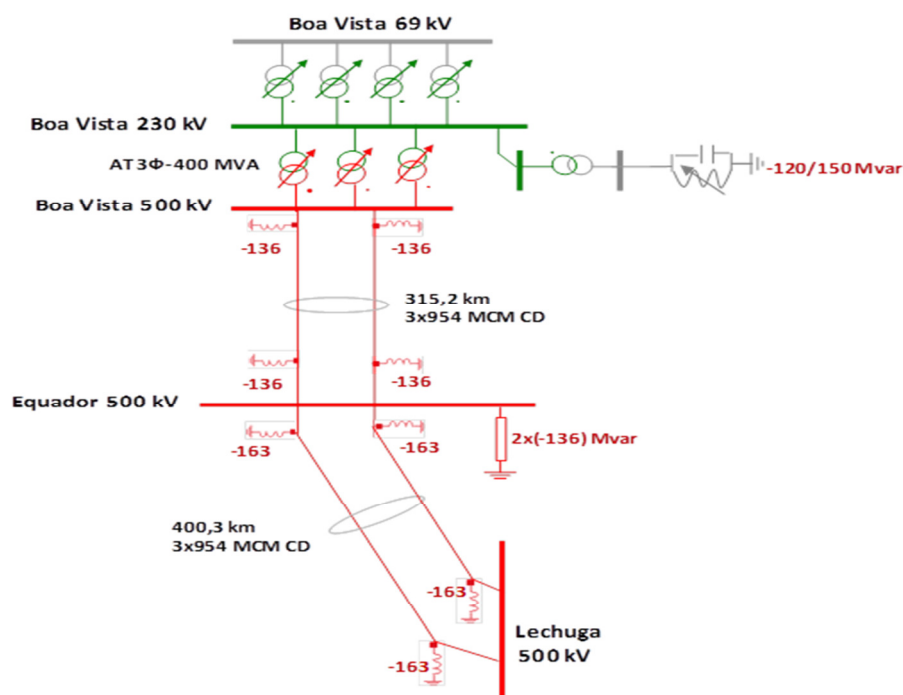
Figura 16 – Interligação Manaus - Boa Vista – Unifilar
