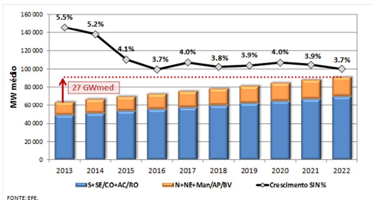
Gráfico 20 – Evolução da carga de energia elétrica no SIN
