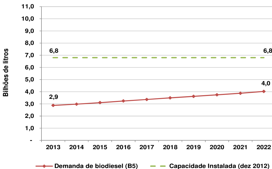
Gráfico 135 – Demanda de biodiesel vs. capacidade instalada
