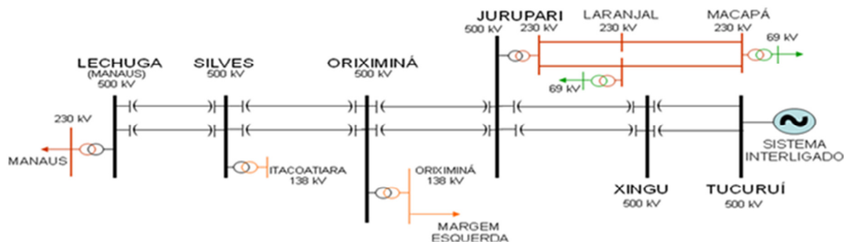
Figura 15 – Interligação Tucuruí-Macapá-Manaus – Unifilar
