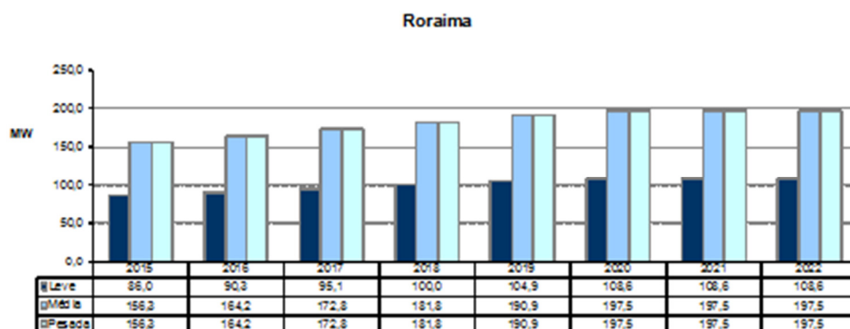
Gráfico 64 – Evolução da carga do Estado de Roraima
