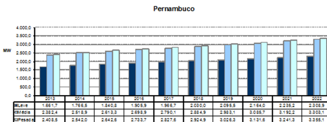
Gráfico 70 – Evolução da carga do Estado de Pernambuco
