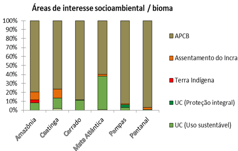
Gráfico 141 – Proporção das interferências da expansão de LT (área da faixa de servidão) com áreas de interesse socioambiental, por bioma
