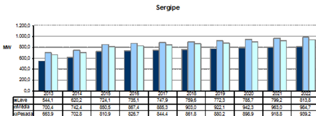
Gráfico 72 – Evolução da carga do Estado de Sergipe
