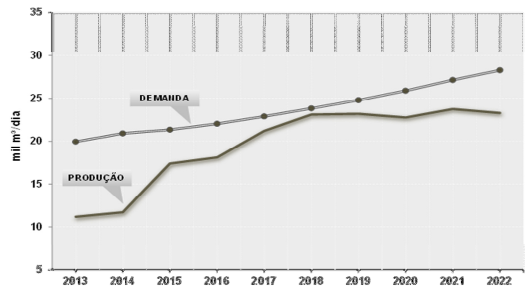
Gráfico 116 – Balanço de coque
