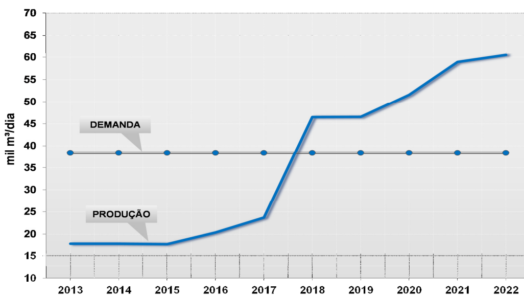
Gráfico 111 – Balanço de nafta
