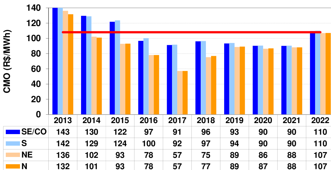
Gráfico 42 – Custo marginal de operação por subsistema
