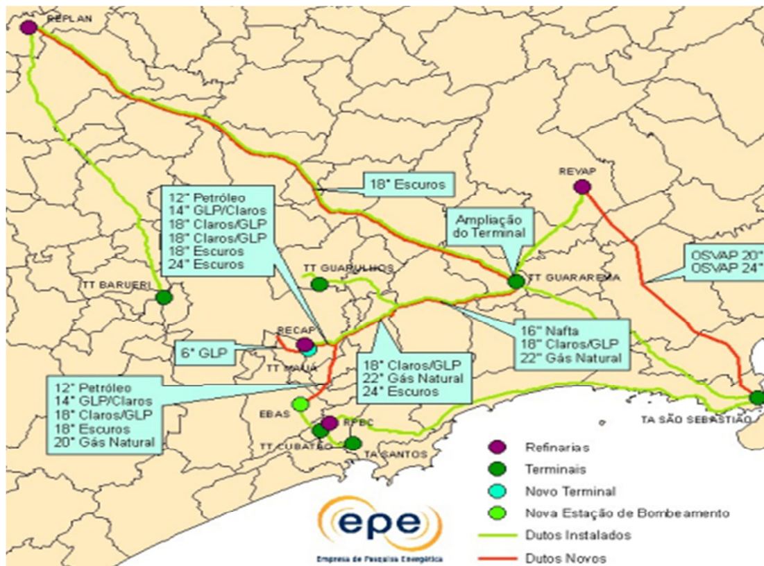
Figura 21 – Situação futura dos dutos de petróleo e derivados do Estado de São Paulo
