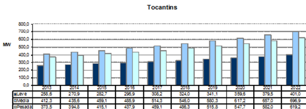
Gráfico 61 – Evolução da carga do Estado do Tocantins
