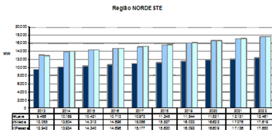
Gráfico 65 – Evolução da carga da Região Nordeste
