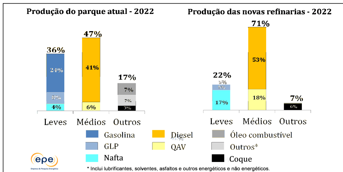
Figura 20 – Perfil de produção das refinarias em 2022
