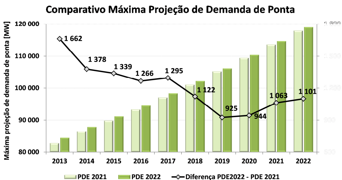
Gráfico 50 – Comparativo da Máxima Projeção de Demanda de Ponta : PDE2022 vs. PDE2021
