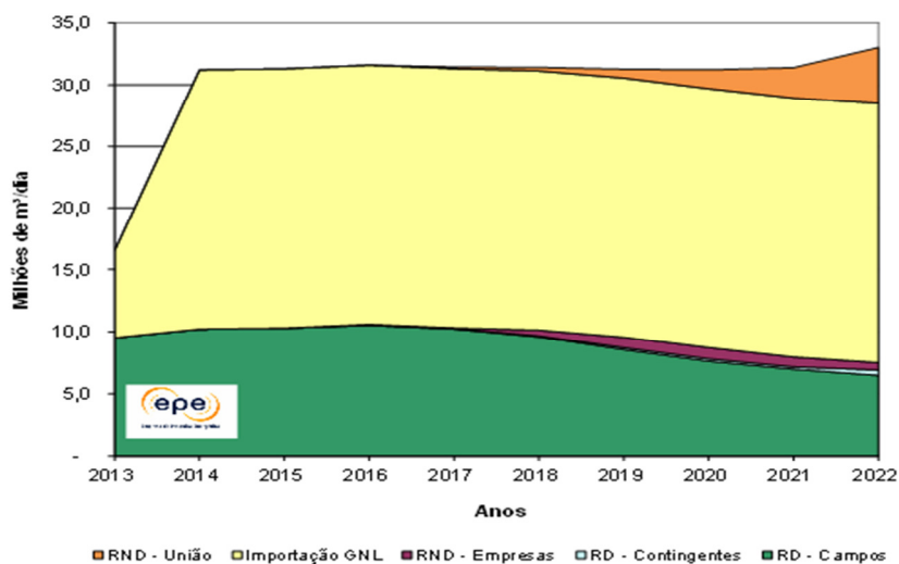
Gráfico 121 – Oferta total para a Região Nordeste
