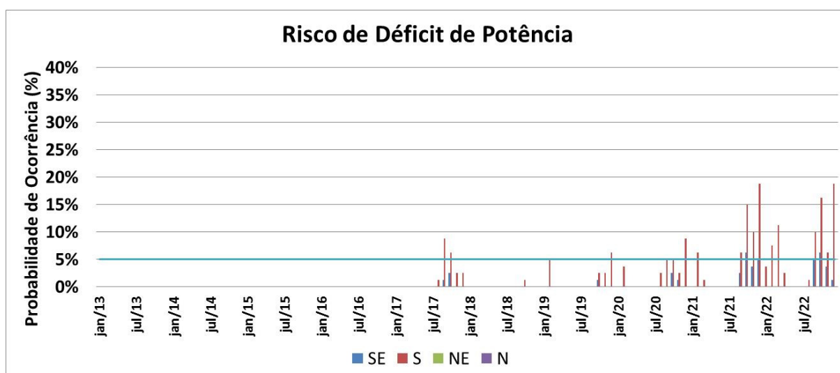
Gráfico 51 – Risco de déficit de potência
