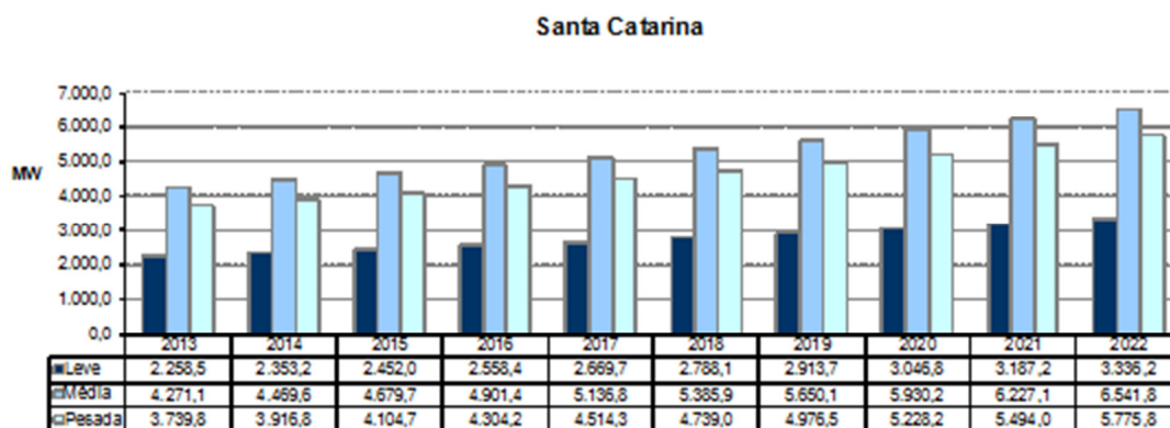
Gráfico 85 – Evolução da carga do Estado de Santa Catarina
