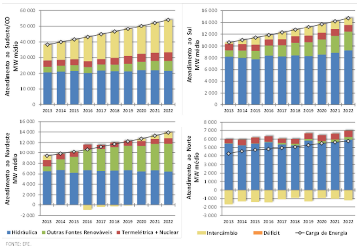
Gráfico 46 – Geração hidrotérmica por subsistema - média dos 2.000 cenários hidrológicos
