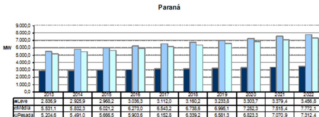
Gráfico 86 – Evolução da carga do Estado do Paraná
