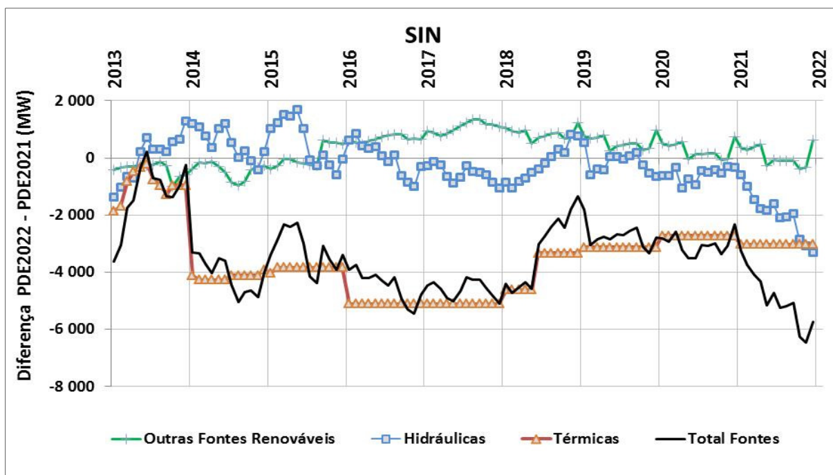
Gráfico 49 – Diferença da disponibilidade de potência (PDE2022 – PDE2021)
