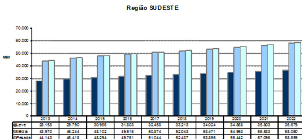
Gráfico 74 – Evolução da carga da Região Sudeste
