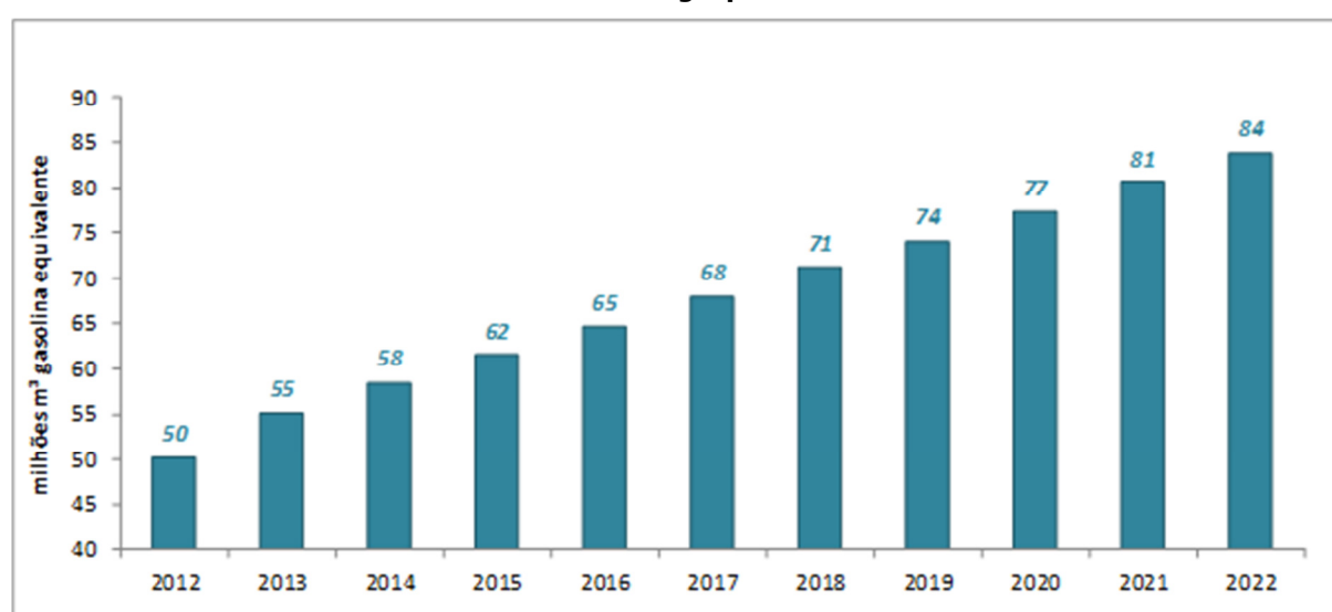
Gráfico 15 – Demanda final de energia para veículos leves do Ciclo Otto
