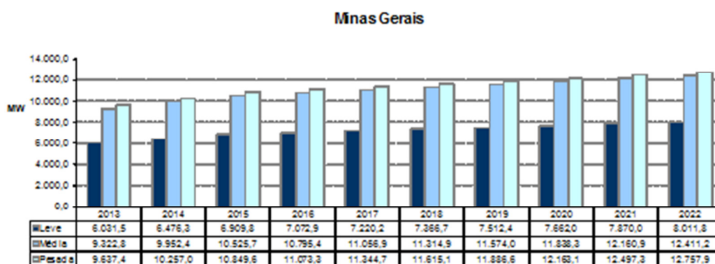
Gráfico 76 – Evolução da carga do Estado de Minas Gerais
